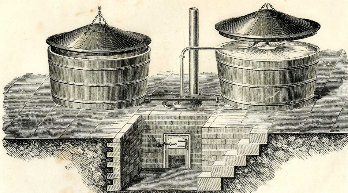
APPAREIL AUTOMOTEUR A LESSIVER PAR ÉBULLITION.
